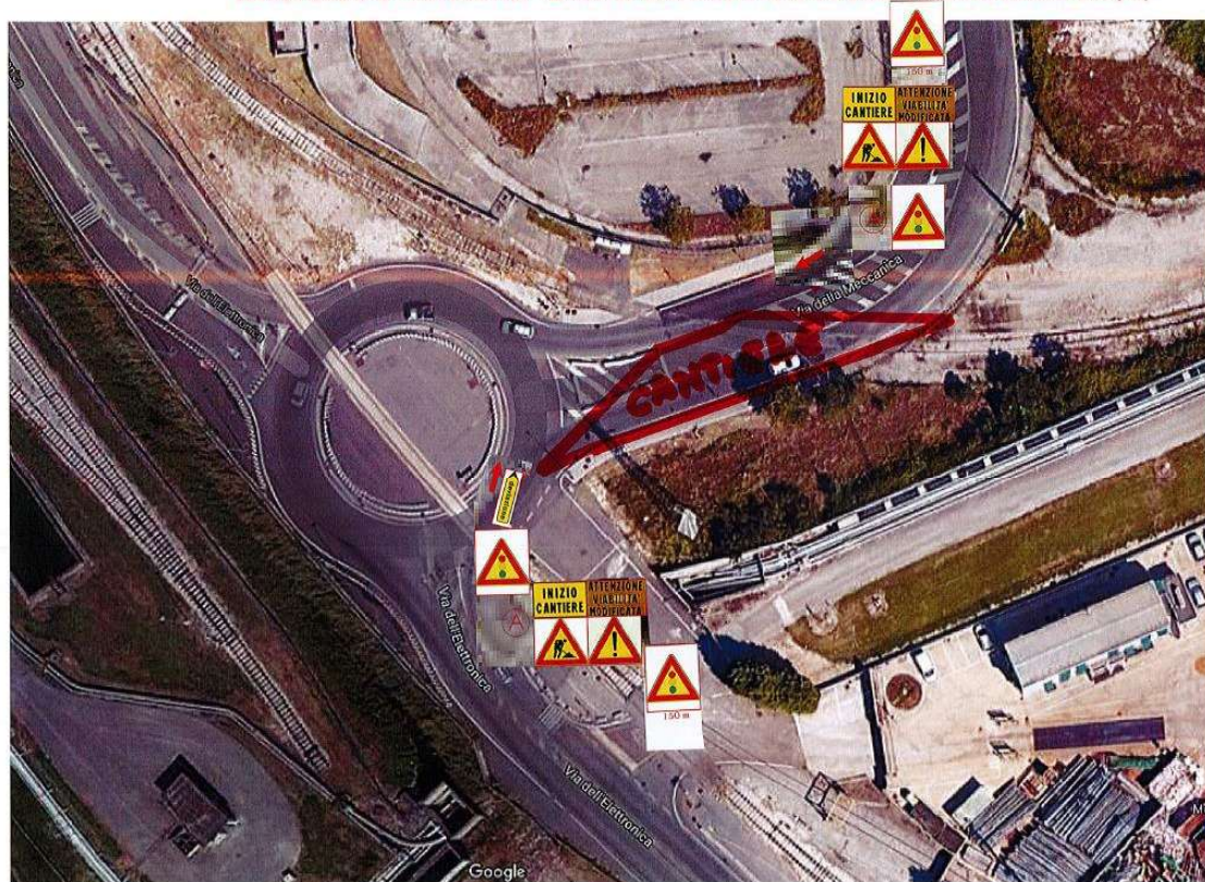
LAYOUT CANTIERE – PLANIMETRIA - LAVORI DI RIFACIMENTO PL SU VIA DELLA MECCANICA MARGHERA (VE)
